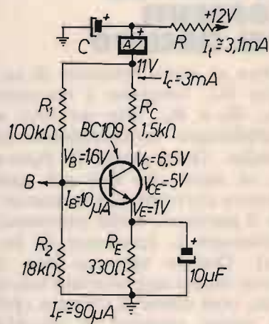
figura 4 Circuito reale di uno stadio a transistor stabilizzato termicamente con partitore sulla base e resistore sull'emettitore. Tutti i valori di tensione e corrente sono stati misurati o calcolati (se il calcolo è più conveniente per una maggiore esattezza).
