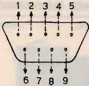
figura 1 Porta joystick C 64: disposizione contatti.
