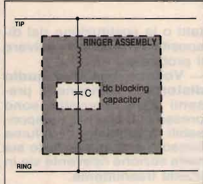
figura 15 Una tipica suoneria dotata di condensatore di blocco per la corrente continua.
