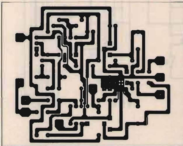
figura 2 Schema del circuito stampato in scala 1:1.
