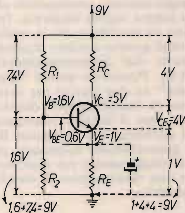
figura 2 Ordine di grandezza delle tensioni in uno stadio con partitore sulla base ( R_1 e R_2 ) e con resistore R_E sull'emettitore. Questo resistore è generalmente bypassato da un condensatore per non diminuire l'amplificazione.
