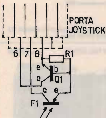
figura 2 Schema elettrico della penna ottica.
