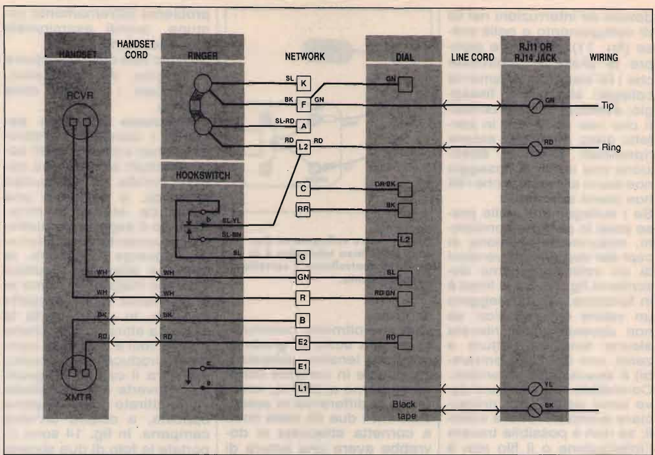
figura 13 Diagramma dei collegamenti di un comune apparecchio telefonico.
