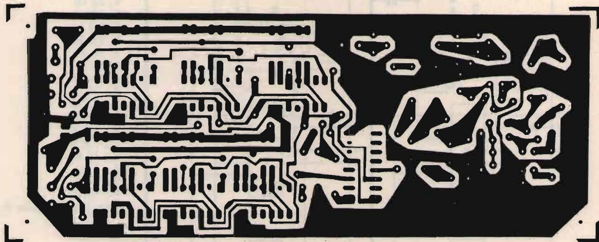
Lato rame.
